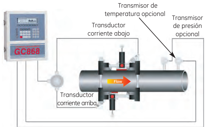
Configuración típica de los medidores para un caudal volumétrico estándar o de masa de vapor
